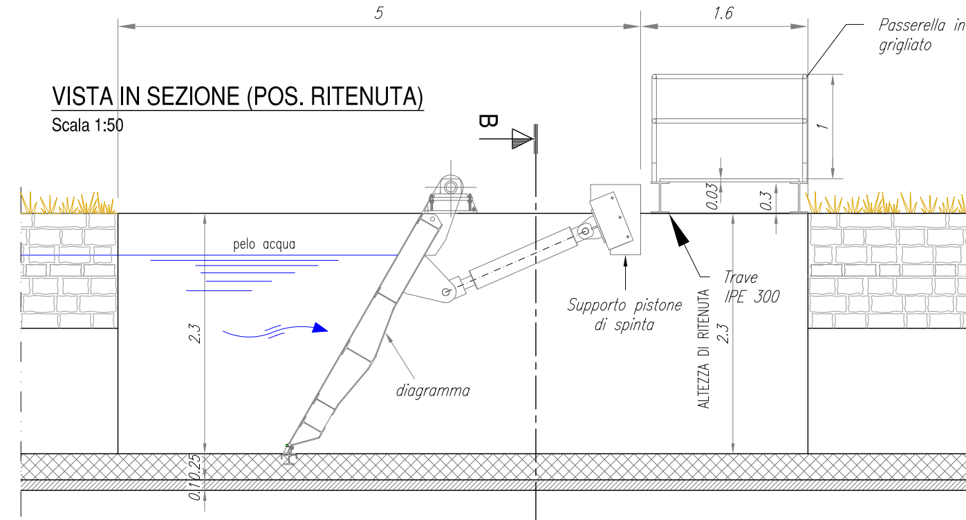
PARATOIA A CLAPE'
