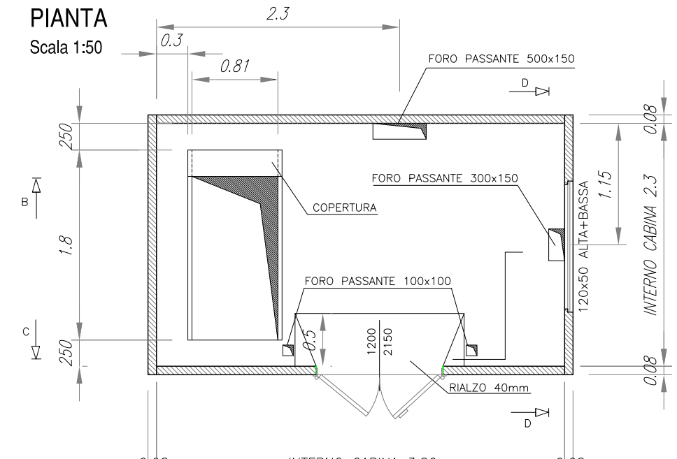
CABINA OMOLOGATA ENEL SOLUZIONE-1
