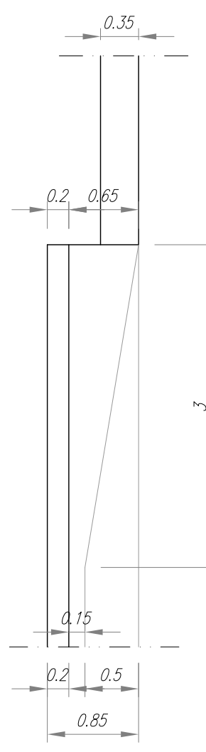
PARTICOLARE RACCORDI TRA SEDIA E MURO Scala 1:50
