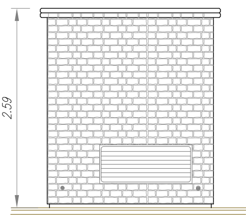
FIANCO DESTRO Scala 1:50
