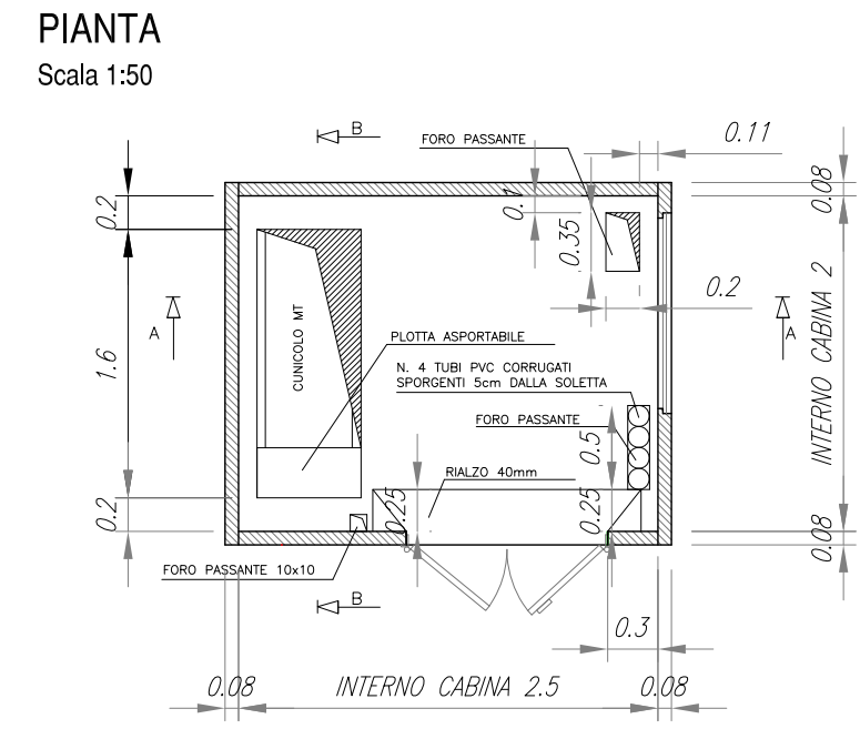
CABINA OMOLOGATA ENEL SOLUZIONE-2
